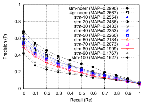
Figura 7: Precisi n vs. Cobertura para las consultas sin corregir (empleando n -gramas).
